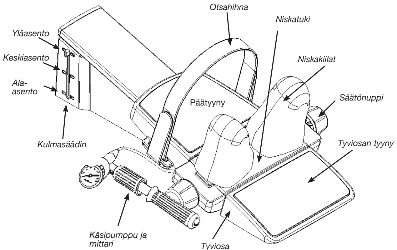
Kuva 1. Saunders-merkkisen kaularangan traktiolaitteen osat
