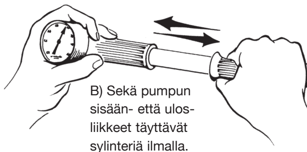
Kuva 3. Käsipumpun käyttäminen
