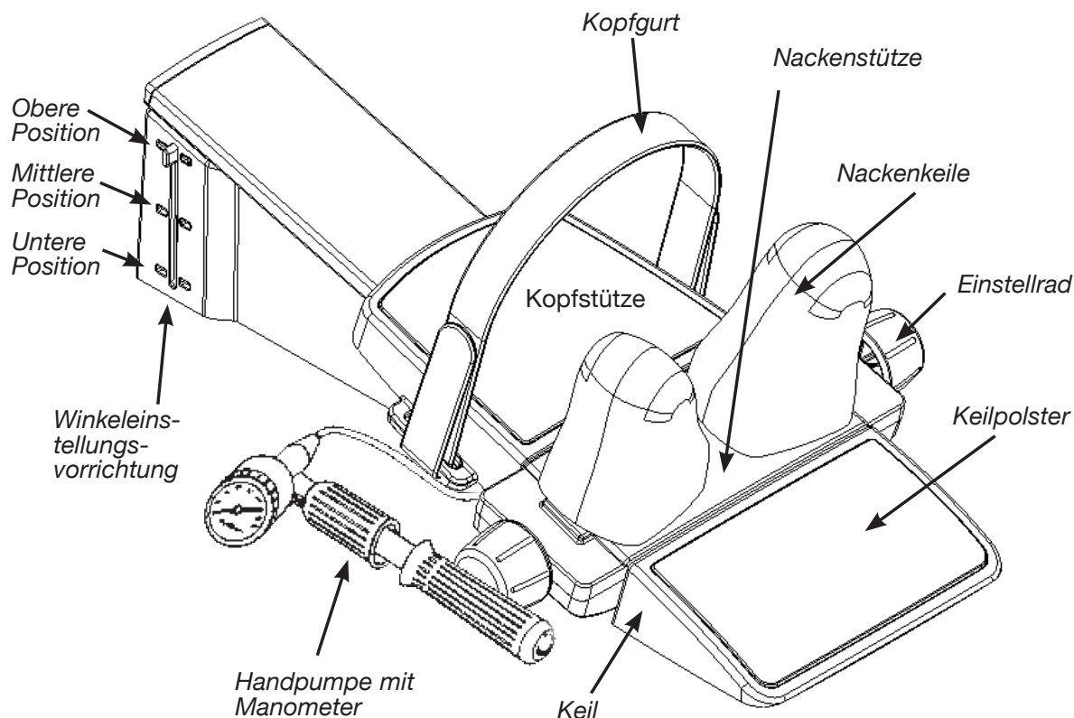
Abbildung 1. Komponenten des Saunders Halswirbelsäulen-Traktionsgeräts
