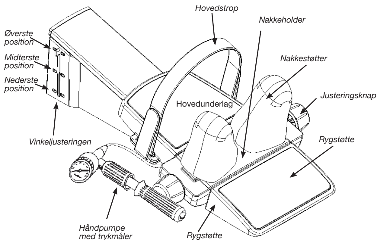
Figur 1. Saunders cervikale traktionsmaskine
