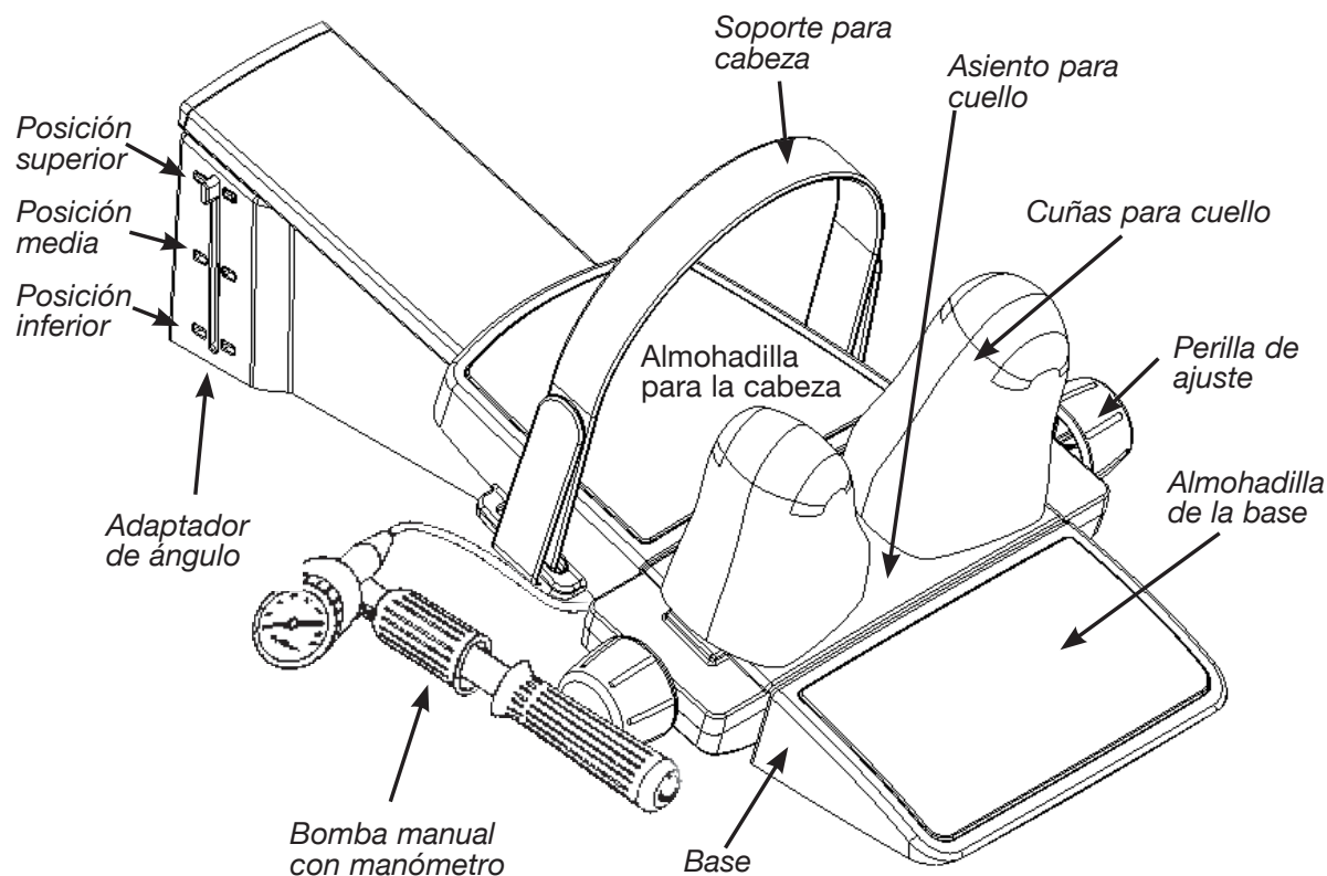
Figura 1. Componentes del dispositivo Saunders tracción cervical
