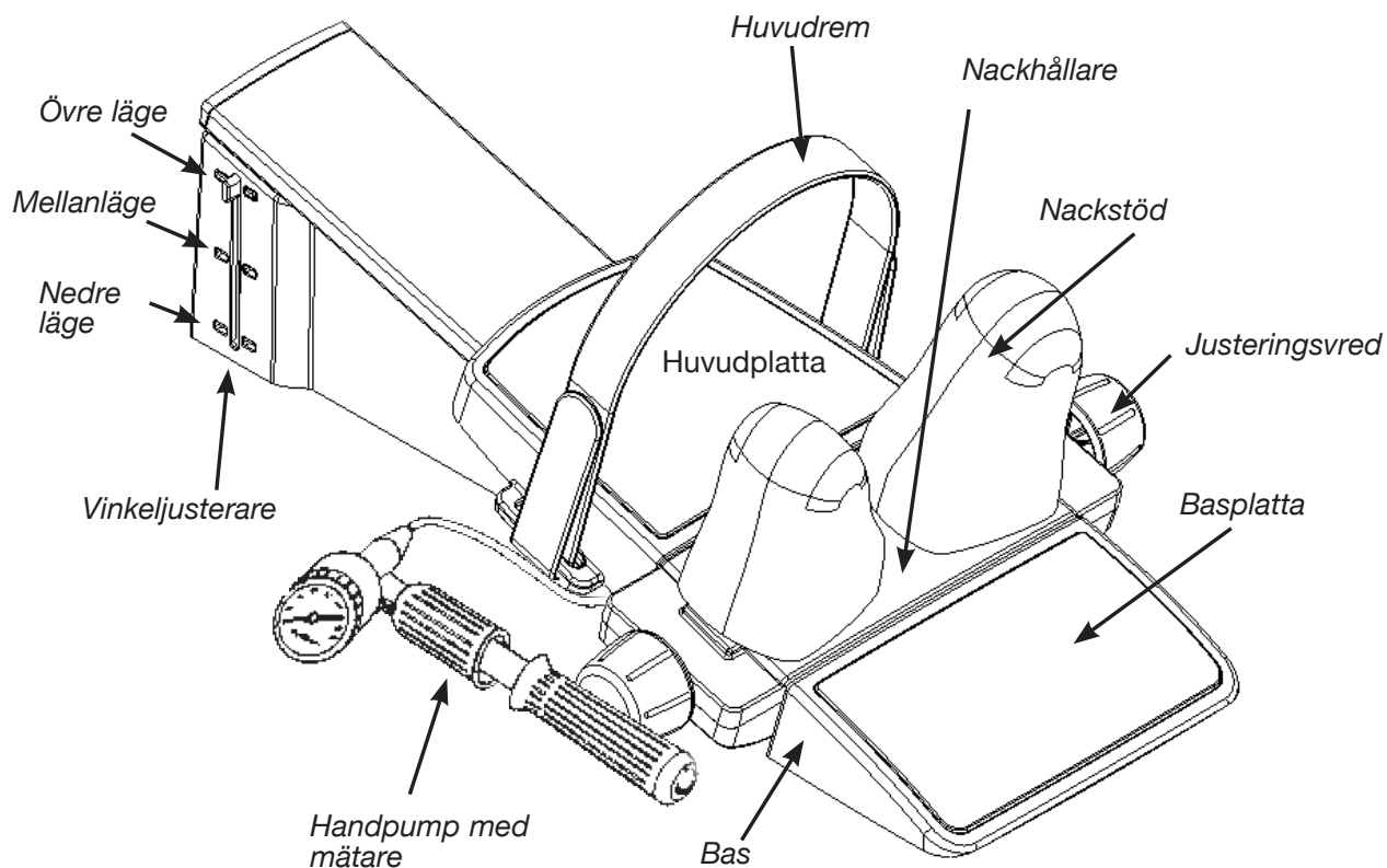
Figur 1. Komponenter i Saunders nacksträckningsapparat
