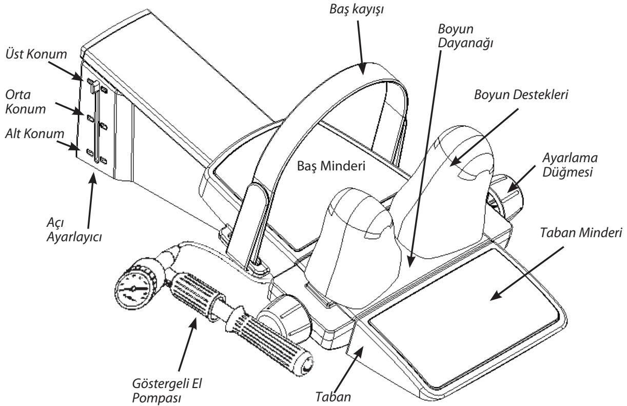
Şekil 1. Saunders Servikal Traksiyon Aygıtının Bileşenleri
