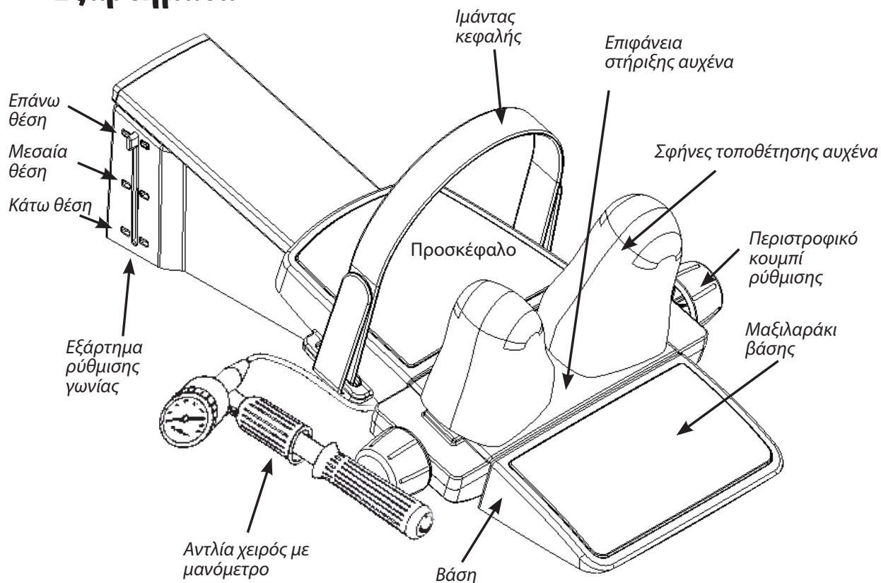
Εικόνα 1. Εξαρτήματα της συσκευής αυχενικής έλξης της Saunders
