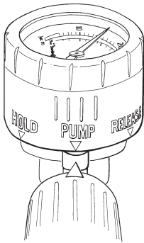
A) Gösterge Yuvasının yakından görünümü.
