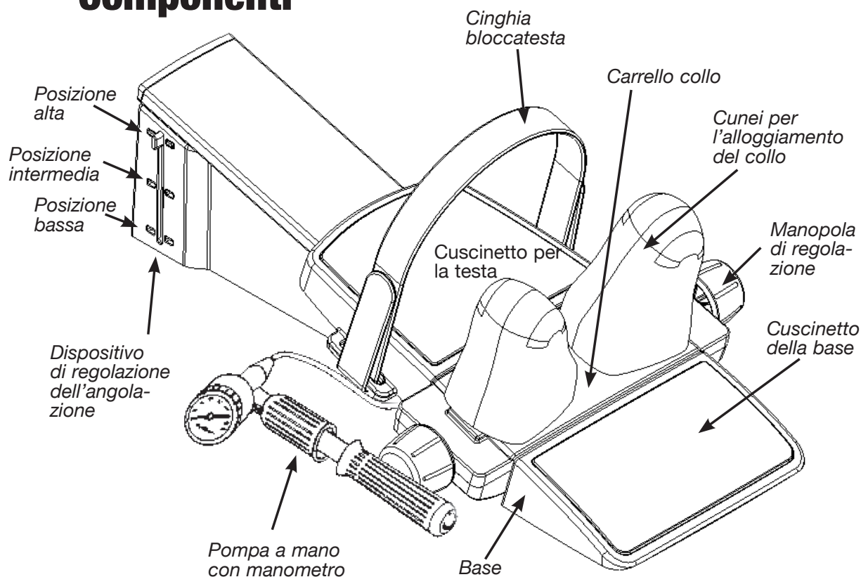
Figura 1. Componenti del dispositivo di trazione cervicale Saunders
