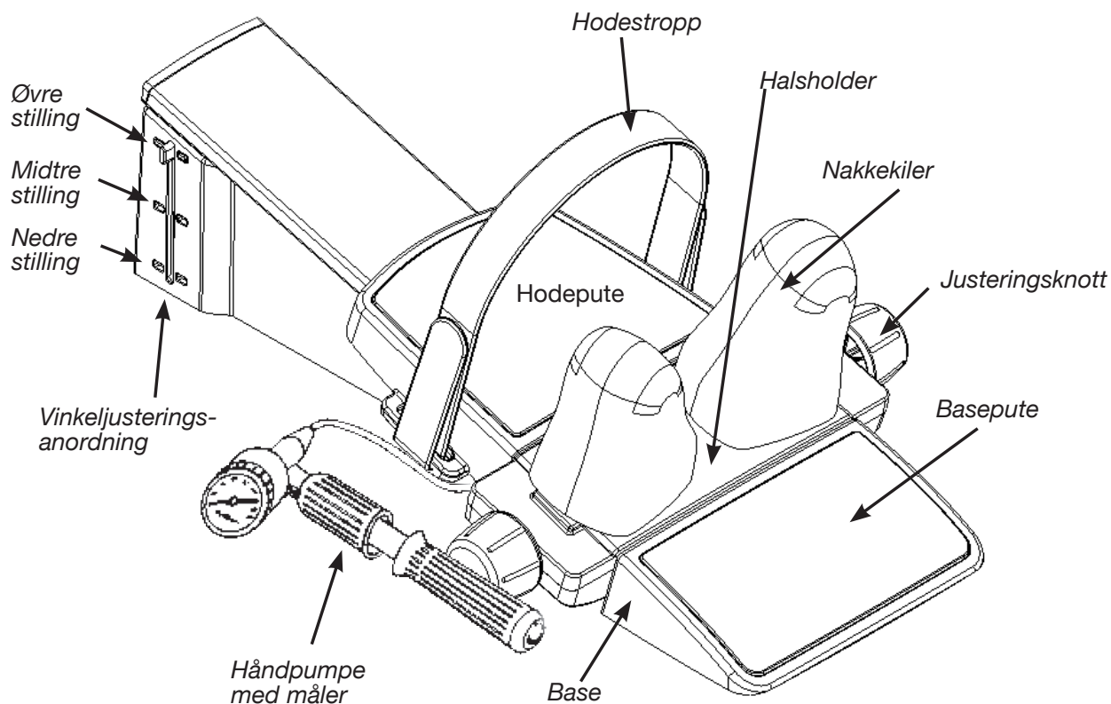
Figur 1. Komponenter i Saunders anordning for cervikal traksjon
